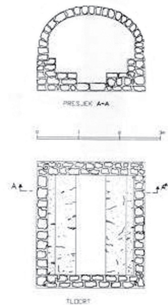
Sl. 6. Grobnica na svod u Previšu, tloris i presjek.
