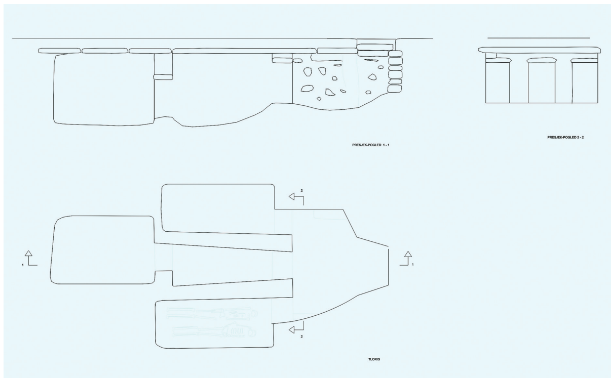
Sl. 8. Tloris kompleksne grobnice u podu katekumeneja.
