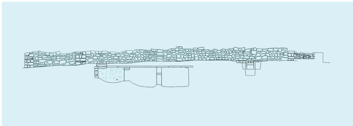
Sl. 7. Kompleksna grobnica u podu katekumeneja (presjek).
