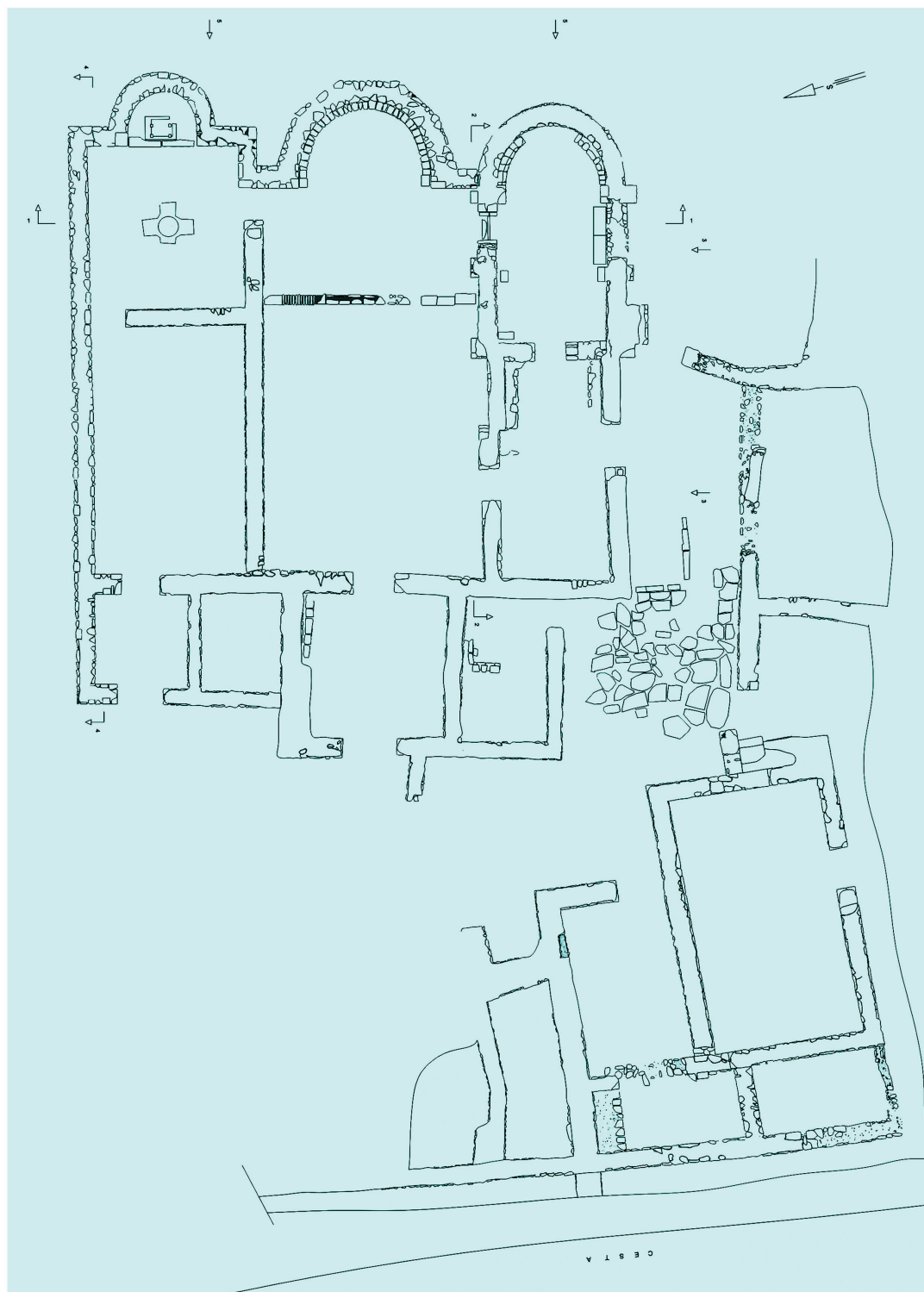
Sl. 2. Tloris otkopane ranokršćanske arhitekture s dijelovima villae rusticae.
