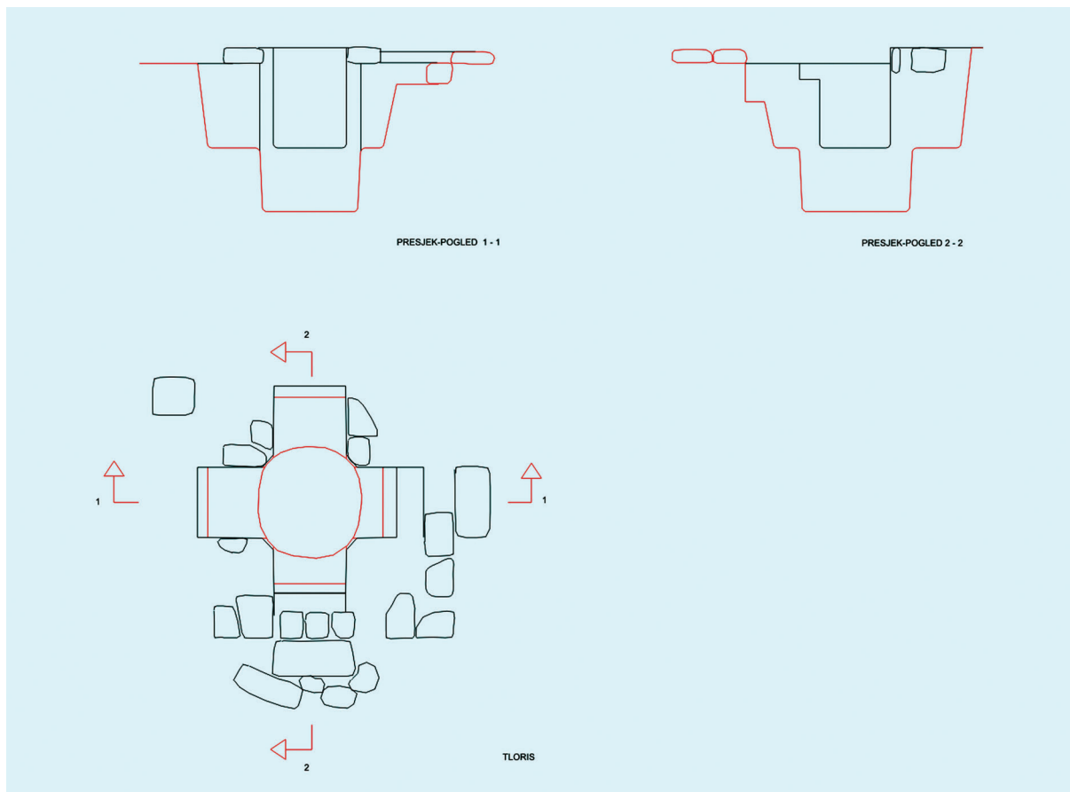
Sl. 6. Tloris krsnog zdenca.
