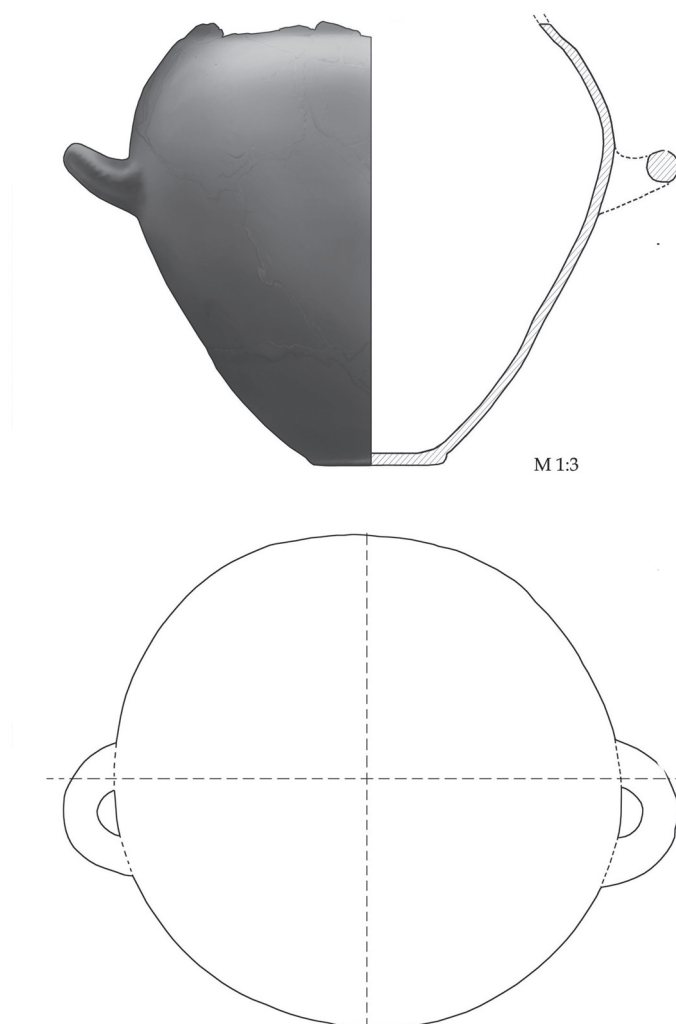
Sl. 17. Nadin, humak 13, grob 4: rekonstruirana keramička žara 2 (crtež: I. Čondić).
