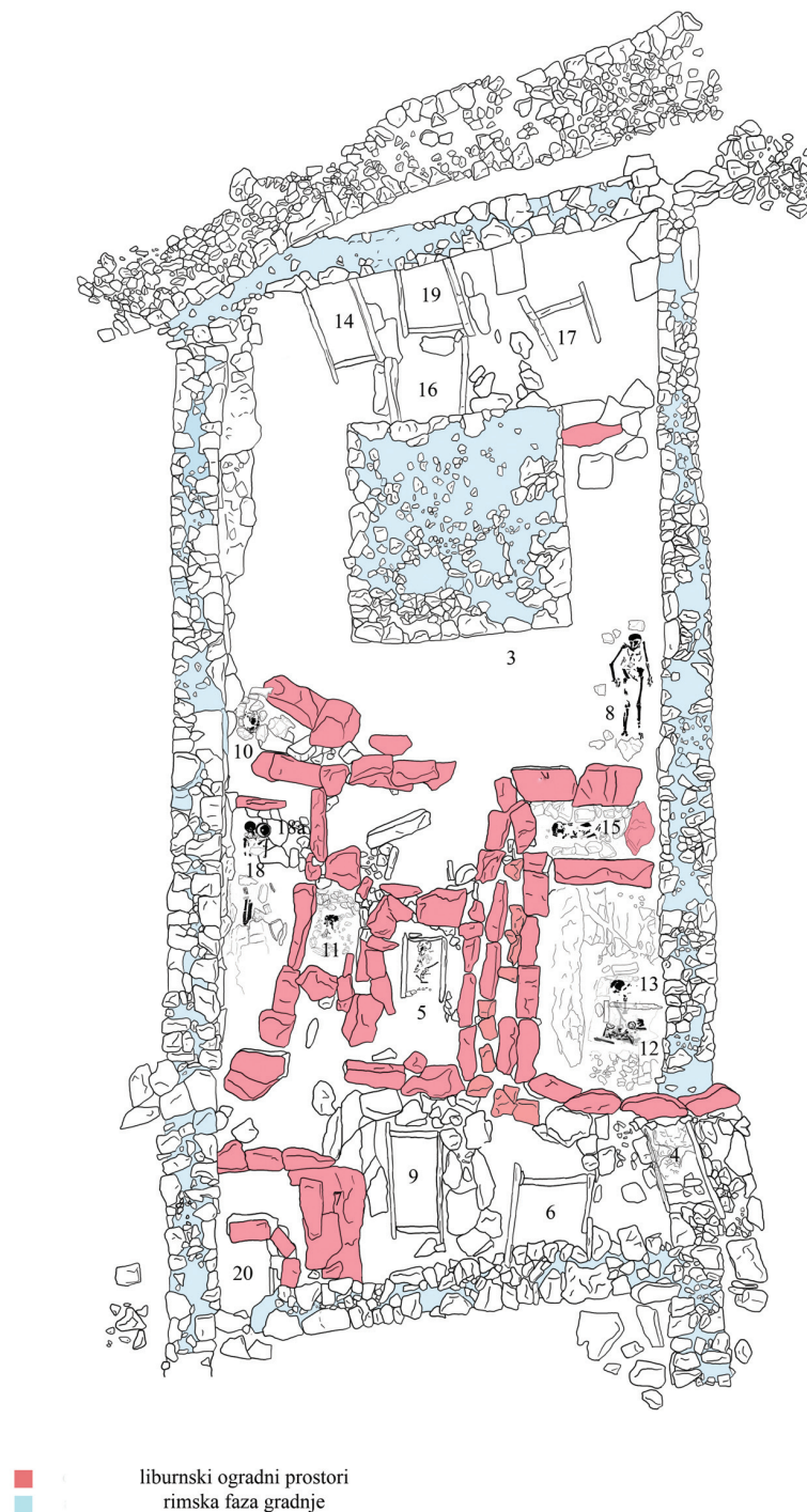
Sl. 24. Nadin, cela I u liburnsko-rimskoj nekropoli: prostorni odnos liburnskih inhumiranih i rimskih spaljenih pokopa (prema S. KUKOČ, 2009).
