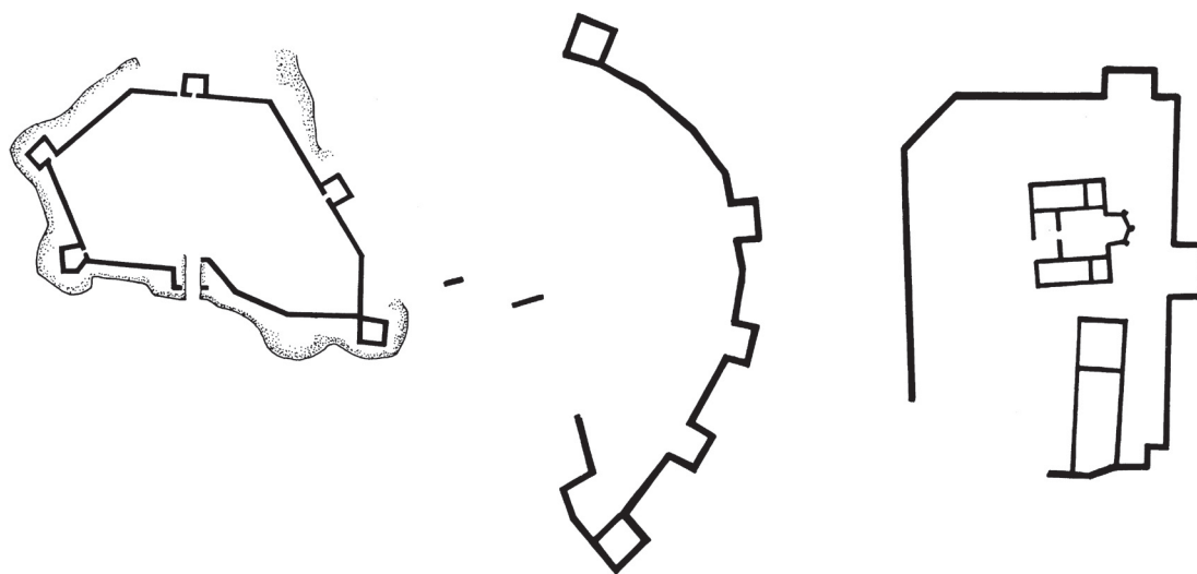
Sl. 8. Gradina Žirje, Vrgada i Osinj. Tlocrti ranobizantskih utvrda (prema GUNJAČA, 1986).
