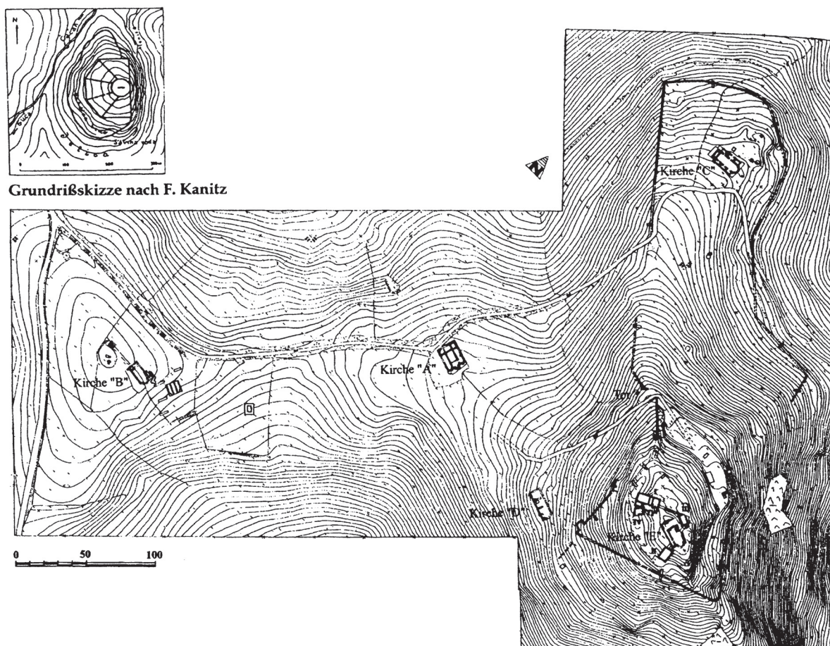
Sl. 2. Gradina Jelica. Plan utvrđenog naselja (prema MILINKOVIĆ, 2008).
