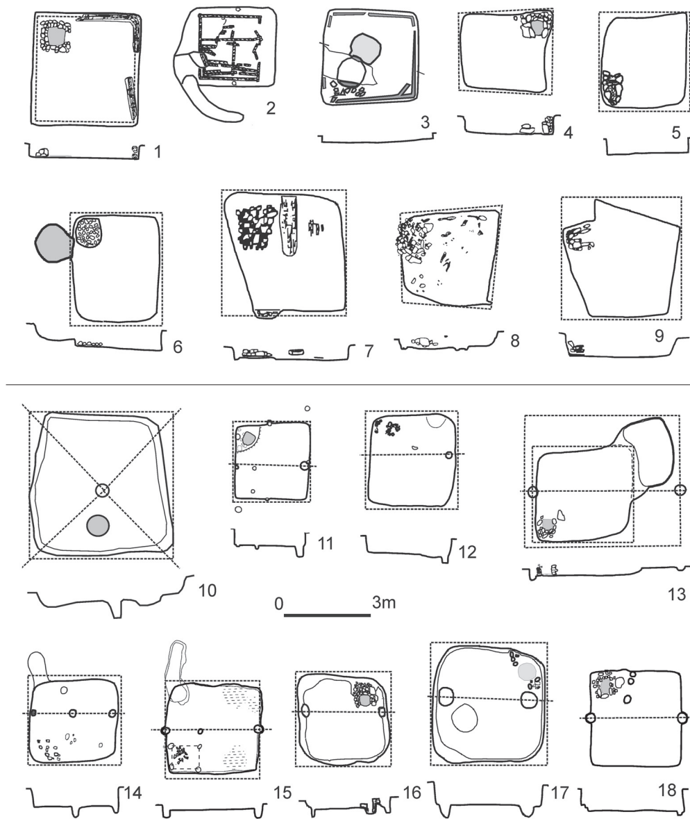
Abb. 1. Quadratische pfostenlose Grubenhäuser und quadratische Grubenhäuser mit Firstsäulenpaar-Zweipostenkonstruktion. 1 – Horodok, Objekt 10; 2 – Volynceve, Objekt 13; 3 – Ložna-Dorohoi, Objekt 1; 4 – Rašків 3, Objekt 82; 5, 6, 12, 14 – Mužla-Čenkov, Objekte 10, 227, 54, 277; 7 – Horodok, Objekt 2; 8 – Žukowice 1, Objekt 18; 9 – Eliseni, Objekt 9; 10 – Zajarje, Objekt 1; 11 – Čataj, Objekt 1; 13, 18 – Břeclav-Pohansko-Lesní školka, Objekte 22, 91; 15 – Štúrovo-Obid, Objekt 8; 16 – Břeclav-Pohansko-Velmožský dvorec, Objekt 86; 17 – Bajč-Vlkanovo, Objekt 10. Fig. 1. Square-shaped pit houses without posts, and square-shaped pit houses – two-pillared construction with pairs of king posts. 1 – Horodok, structure 10; 2 – Volynceve, structure 13; 3 – Ložna-Dorohoi, structure 1; 4 – Rašків 3, structure 82; 5, 6, 12, 14 – Mužla-Čenkov, structure 10, 227, 54, 277; 7 – Horodok, structure 2; 8 – Žukowice 1, structure 18; 9 – Eliseni, structure 9; 10 – Zajarje, structure 1; 11 – Čataj, structure 1; 13, 18 – Břeclav-Pohansko-Lesní školka, structure 22, 91; 15 – Štúrovo-Obid, structure 8; 16 – Břeclav-Pohansko-Velmožský dvorec, structure 86; 17 – Bajč-Vlkanovo, structure 10.
