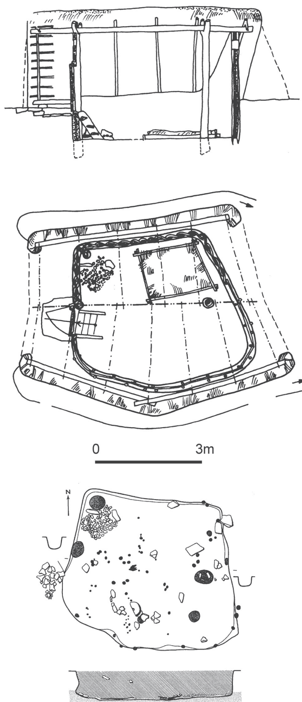
Abb. 8. Rekonstruktion von Vielpostengrubenhäusern mit Flechtwerkwänden 1 – Březno, Obj. 5 (nach I. Pleinerová). Fig. 8. Reconstruction of multi-pillared pit houses with wattle and daub walls 1 – Březno, structure 5 (after I. Pleinerová).
