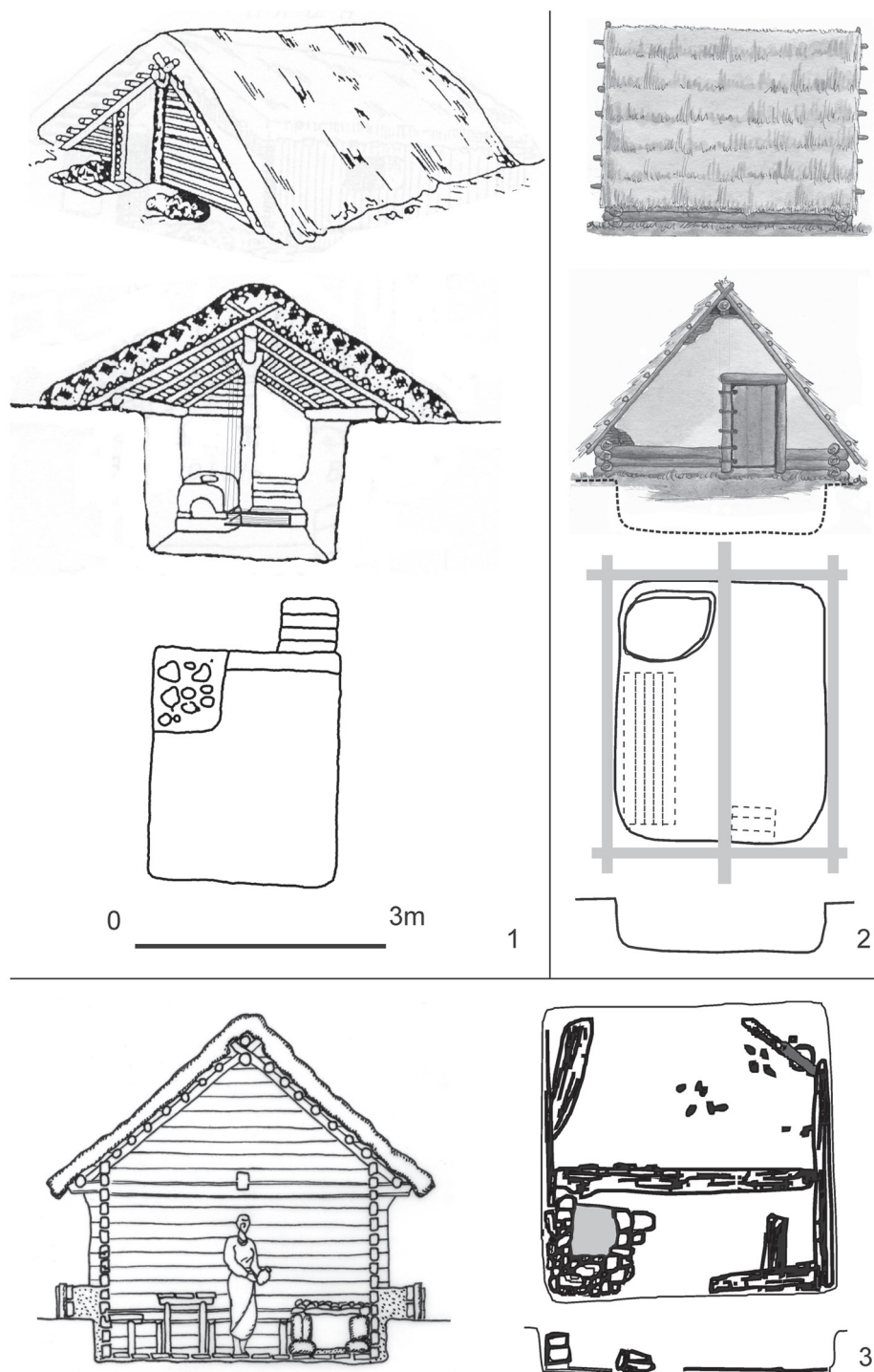
Abb. 5. Rekonstruktionen quadratischer pfostenloser Grubenhäuser (Blockbaugrubenhäuser). 1 – Kaniw (nach G. G. Mezenceva), 2 – Šurany-Nitriansky Hrádok, Objekt 9 (nach P. Šalkovský); 3 – Raškiev 3, Objekt 50 (nach V. D. Baran). Fig. 5. Reconstructions of square-shaped pit houses without posts (block-construction pit houses). 1 – Kaniw (after G. G. Mezenceva), 2 – Šurany-Nitriansky Hrádok, structure 9 (after P. Šalkovský); 3 – Raškiev 3, structure 50 (after V. D. Baran).
