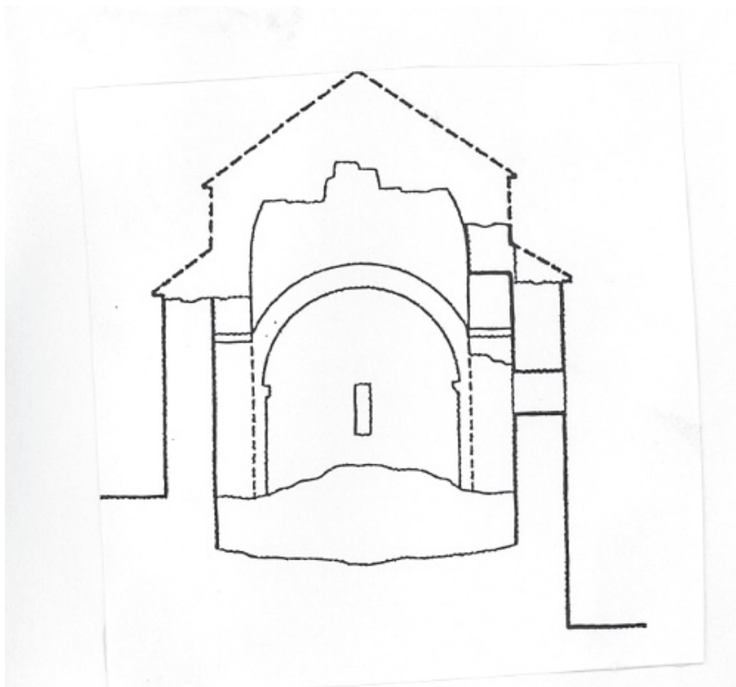
Sl. 7. Sv. Nikola na otoku Sušcu, presjek (prema Domančiću).
