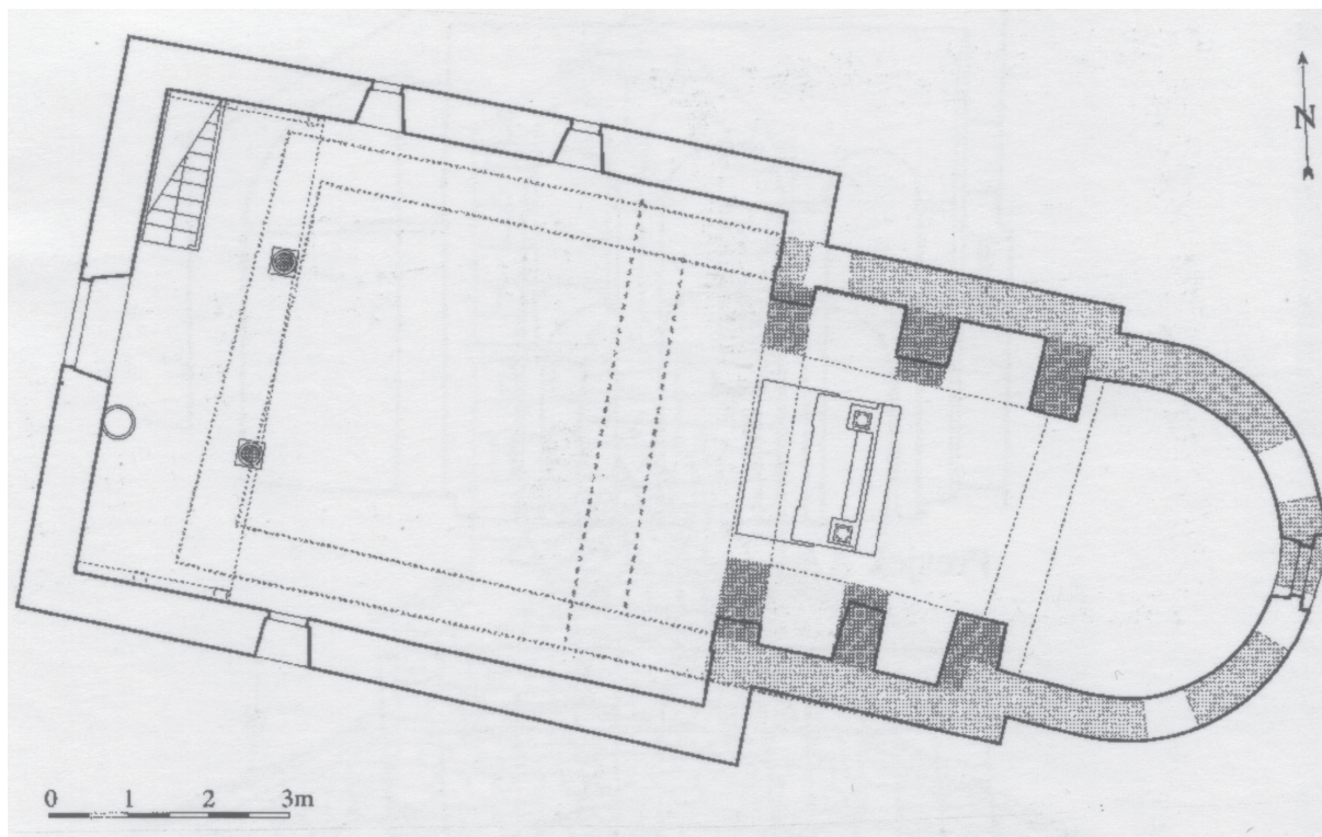
Sl. 3. Sv. Stjepan u Pučišćima na Braču, tlocrt s označenim slojevima (prema R. BUŽANČIĆ, 1994).
