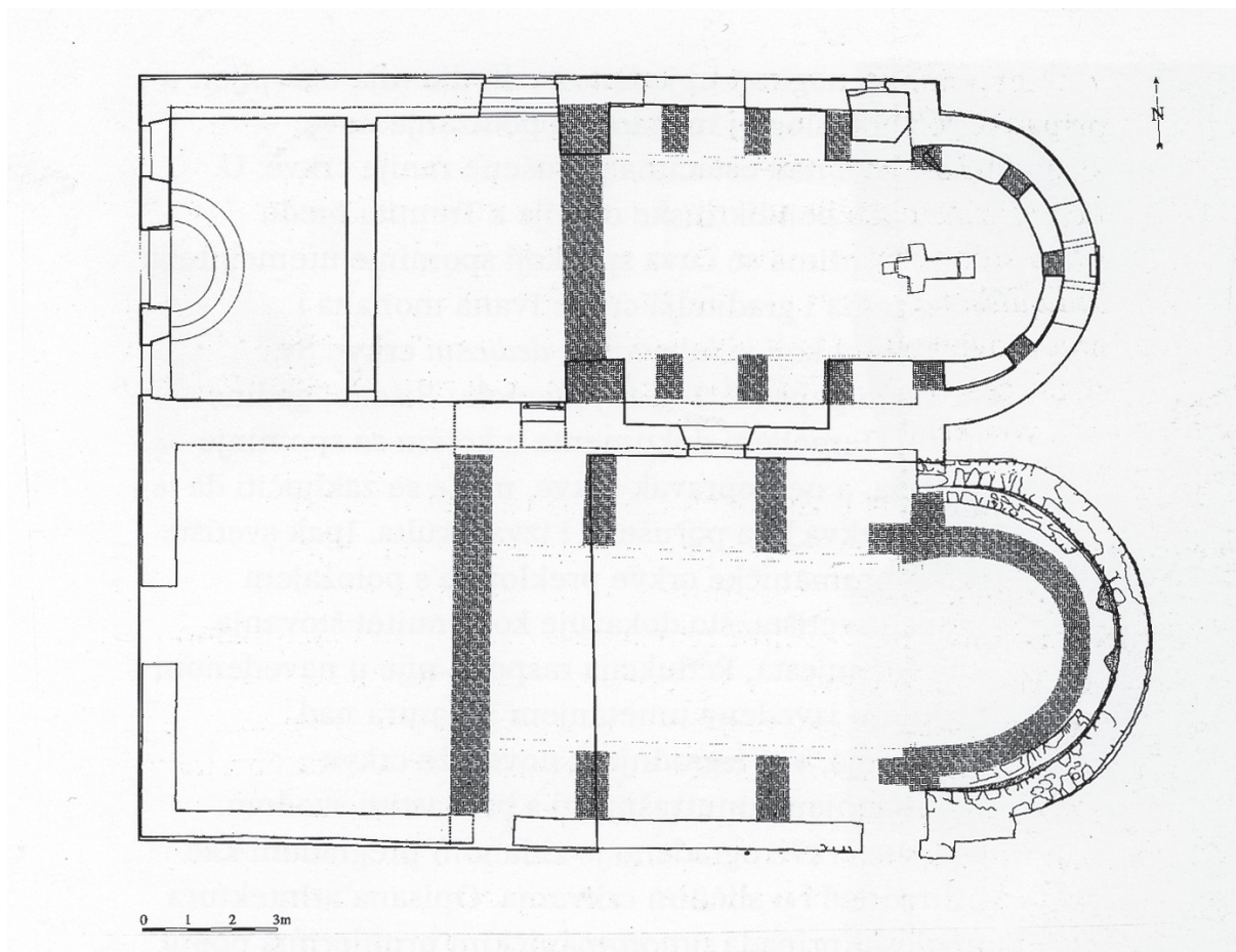
Sl. 6. Dvojne crkve u Starom Gradu, tlocrt s označenim slojevima (prema R. BUŽANČIĆ, 1996). Sjeverna crkva je Sv. Marija, a južna Sv. Ivan Krstitelj.
