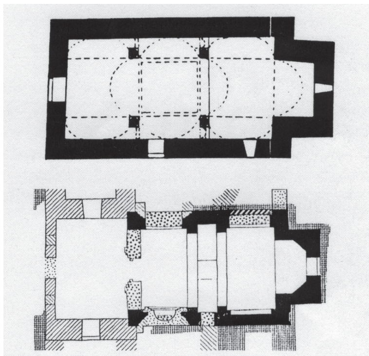
Sl. 12. Usporedni tlocrti Sv. Mikule u Splitu (prema T. Marasoviću) i Sv. Petra u Bijelom polju (prema J. Neškoviću).
