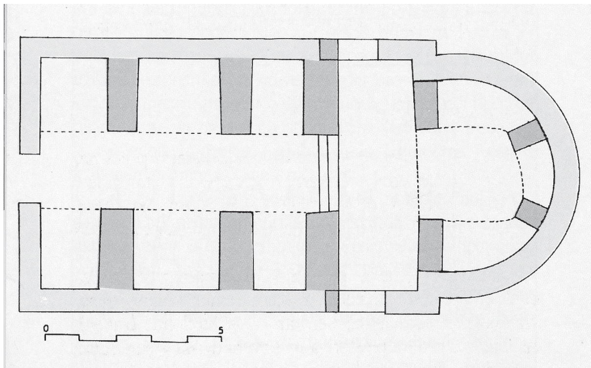
Sl. 8. Sv. Andrija u Baćini, tlocrt s označenim slojevima (prema T. MARASOVIĆ, 1998).
