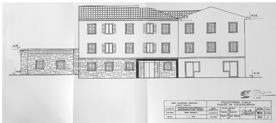
Slika 1. Nacrt zgrade Sabirnog arhivskog centra u Novalji iz dokumentacije fonda HR-DAZD-SACN-3 Upravni odjel za graditeljstvo, UP/I-361-03/05-01/117, mapa 246.
