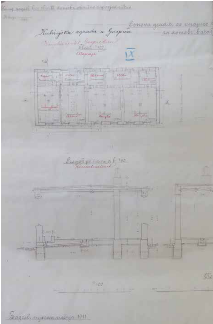
Sl. 8. Kuhinjska zgrada u Gospiću, 1911., Gustav Schmid (HR-HDA, Fond 466, Vojno-građevinski odjel XIII. zbornice, kut. 5)
