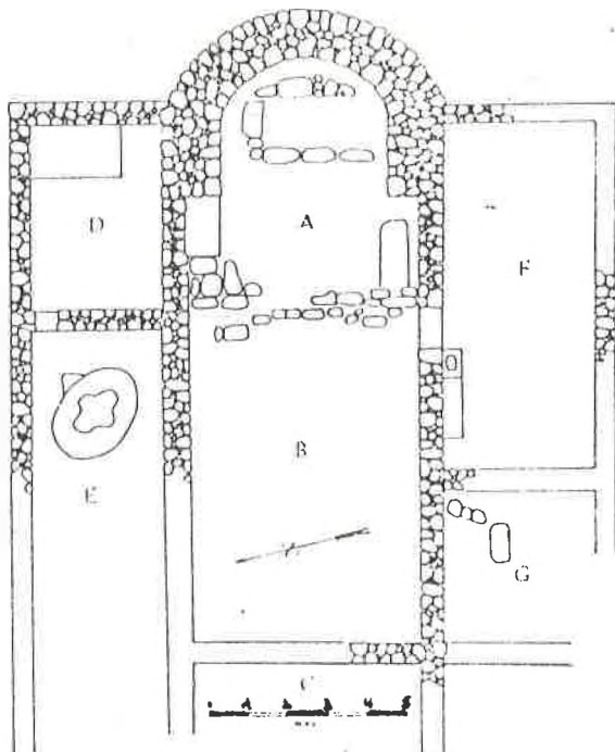
Sl. 6. Tlocrt crkve u Klobuku (prema: Đ. Basler).
