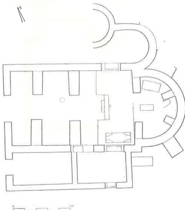
Sl. 12. Tlocrt crkve u Sladincu - Bačina kod Kardeljeva (prema: I. Fisković).
