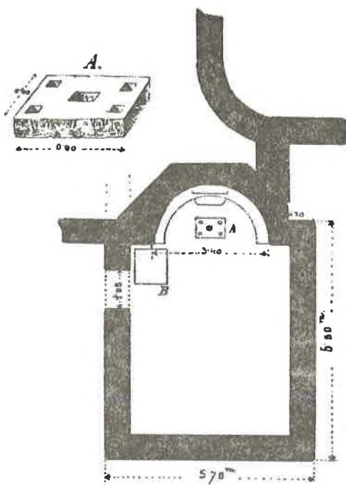
Sl. 11. Tlocrt crkve u Borasima (prema: Č. Truhelka).
