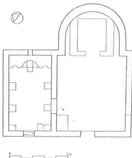
Sl. 14. Tlocrt crkve sv. Petra kod Stona (prema: I. Fisković).
