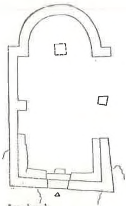
Sl. 16. Tlocrt crkvice na Lučnjaku (prema: I. Fisković).
