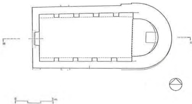
Sl. 15. Tlocrt crkve sv. Ivana kod Stona (prema: I. Fisković).
