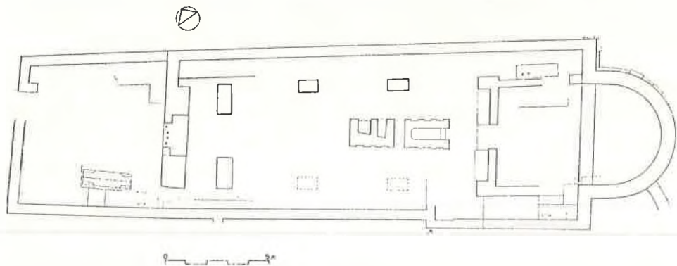
Sl. 13. Tlocrt crkve sv. Mandaljene u Stonskom polju (prema: I. Fisković).
