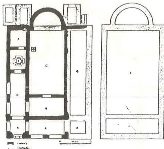
Sl. 4. Tlocrt dvojnih bazilika u Mogorjelu (prema: Đ. Basler).
