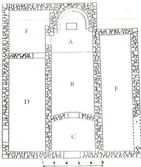
Sl. 8. Tlocrt crkve u Docima (prema: Đ. Basler).
