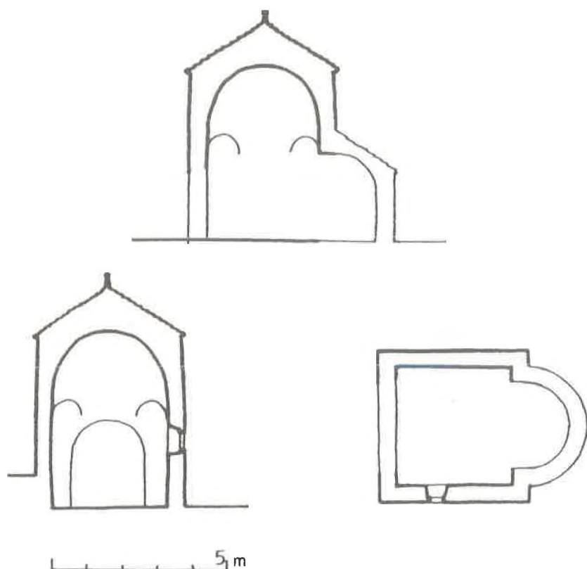
Sl. 4. Poprečni i uzdužni presjek i tloris Crkve Sv. Pelegrina u Savru (P. Vežić). Fig. 4. The transversal and longitudinal cross-section and ground plan of the church of St Pelegrin in Savar (P. Vežić).
