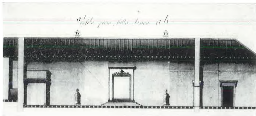
Nacrt uređenja Vijećnice, presjek, 1816. godina
