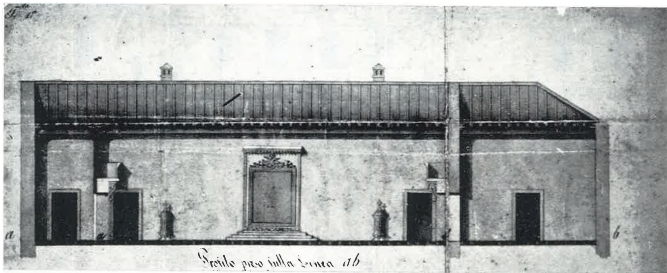
Nacrt uređenja Vijećnice, presjek, 1817. godina
