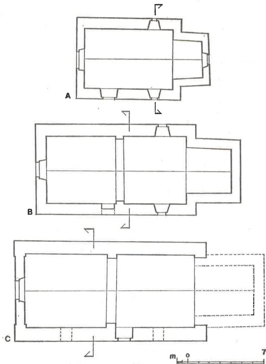
Tlocrni crkava: A. Kula Atagića, B. Zaglav, C. Sali
