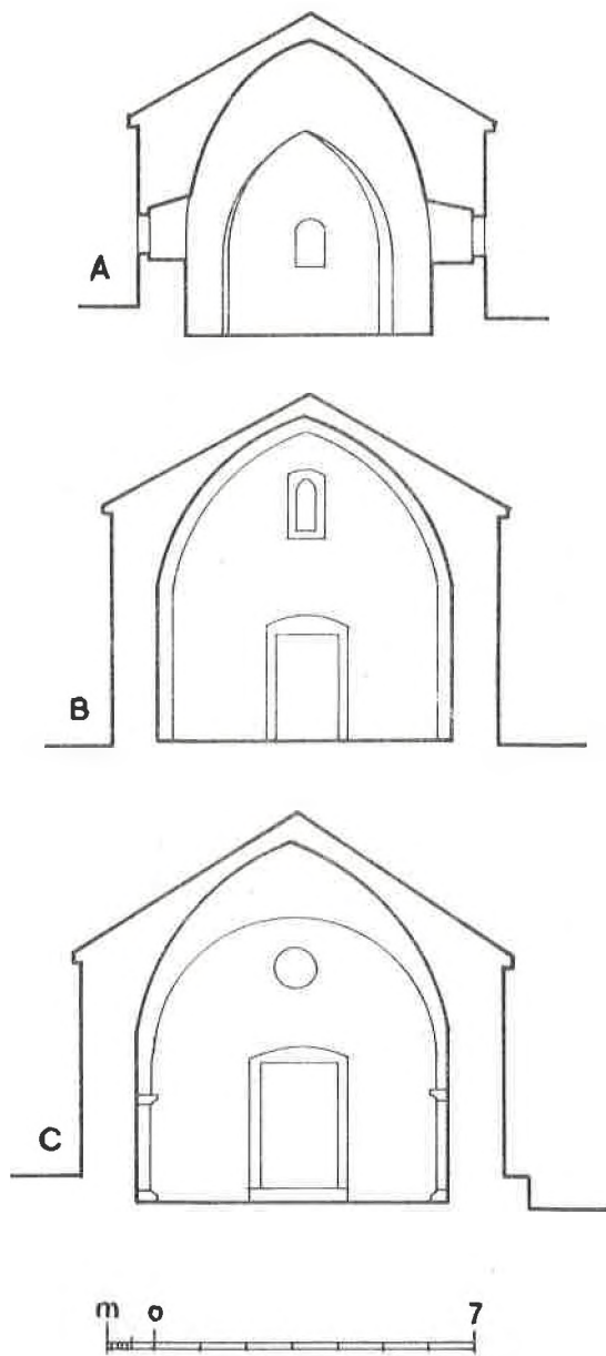
Poprečni presjeci crkava: A. Kula Atlagića, B. Zaglav, C. Sali
