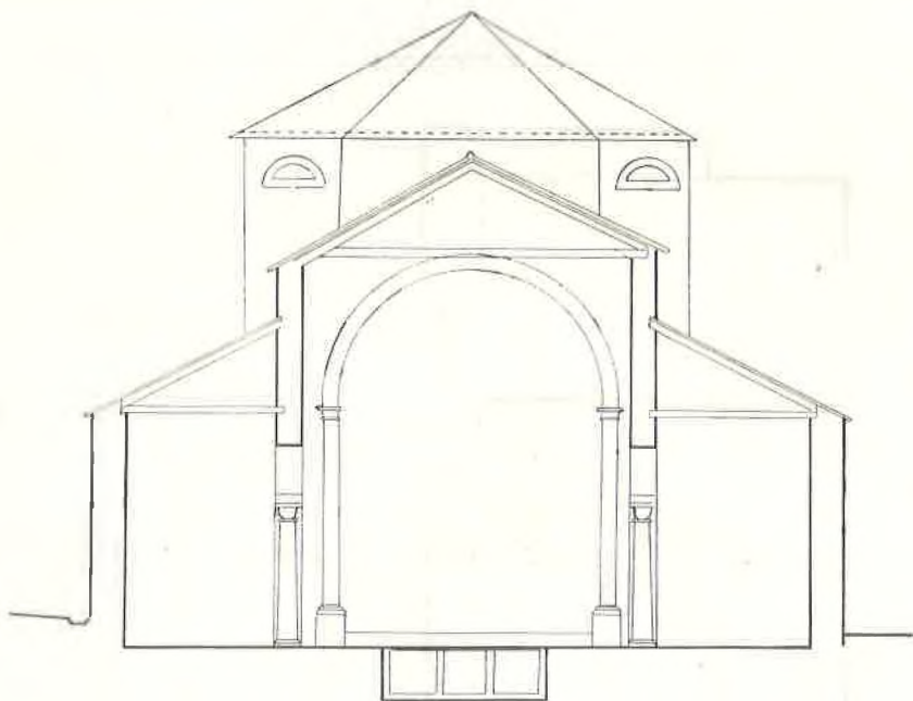
Sl. 4. Poprečni presjek crkve sv. Tome po Hatzingerovu nacrtu. Fig. 4. Spaccato trasversale della chiesa di S. Tomaso dal disegno del Hatzinger.
